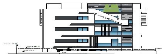
ΒΟΡΕΙΟΔΥΤΙΚΗ ΟΨΗ ΚΤΗΡΙΟΥ Β' ΚΛΙΜΑΚΑ 1/200
