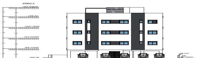
ΤΟΜΗ - ΟΨΗ Κ/Α' ΚΛΙΜΑΚΑ 1/200
