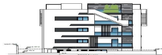
ΒΟΡΕΙΟΔΥΤΙΚΗ ΟΨΗ ΚΤΗΡΙΟΥ Β' ΚΛΙΜΑΚΑ 1/200
