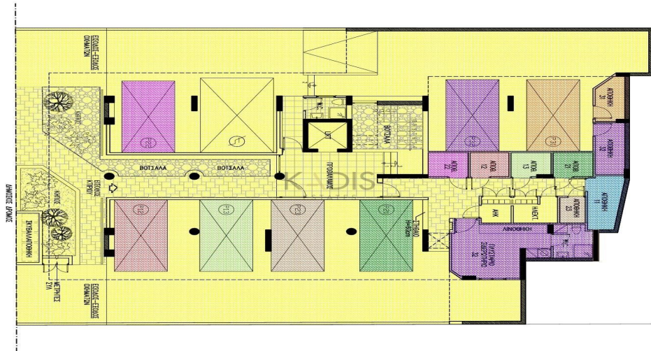
ΟΡΙΖΟΝΤΙΟΣ ΔΙΑΧΩΡΙΣΜΟΣ κατόψη Υποστέγου
