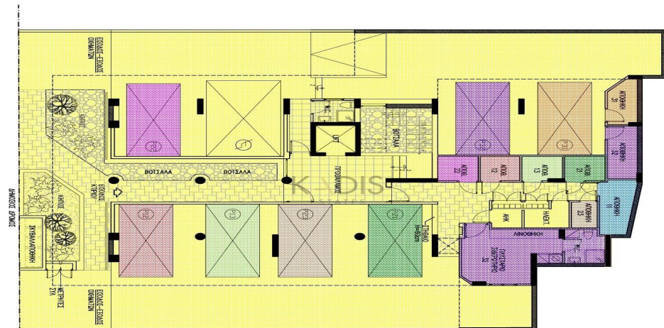
ΟΡΙΖΟΝΤΙΟΣ ΔΙΑΧΩΡΙΣΜΟΣ κατόψη Υποστέγου
