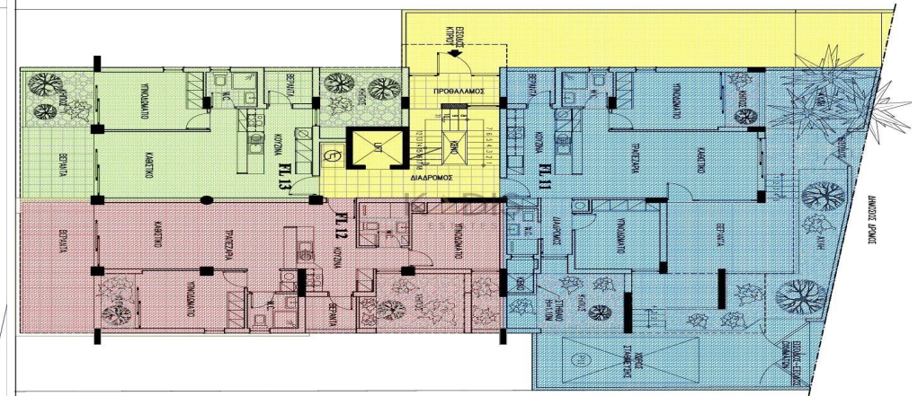
ΟΡΙΖΟΝΤΙΟΣ ΔΙΑΧΩΡΙΣΜΟΣ κατόψη 1ου Ορόφου
