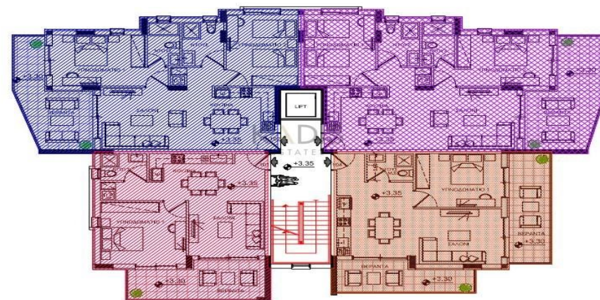
ΚΑΤΟΨΗ 1ου ΟΡΟΦΟΥ - ΔΙΑΧΩΡΙΣΜΟΣ ΚΑΙΜΑΚΑ 1:100
