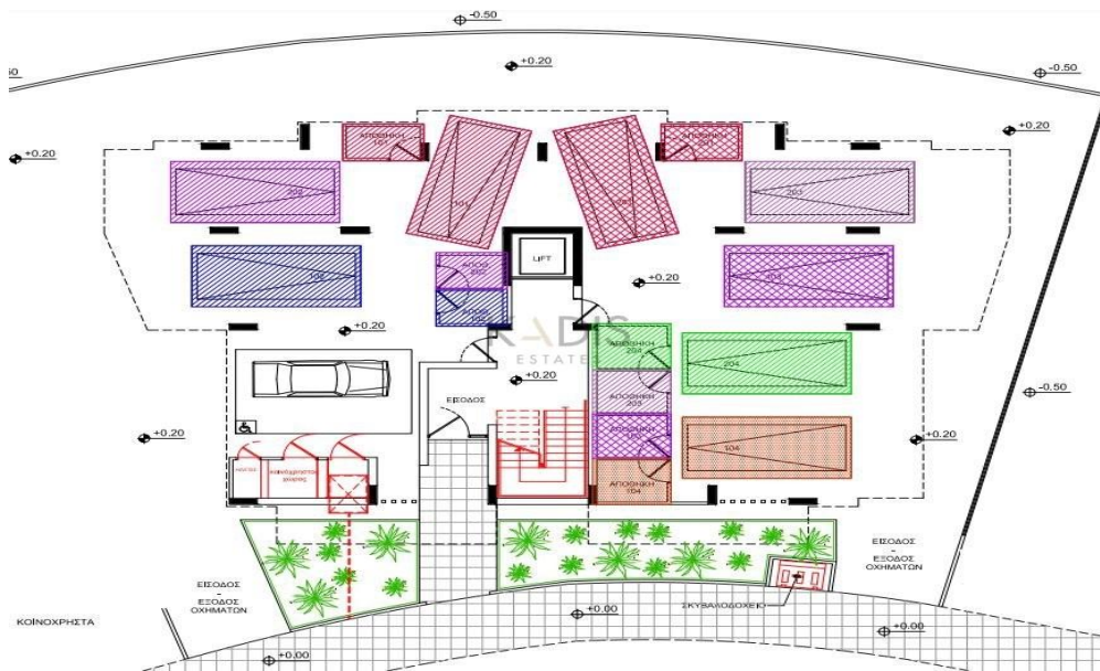
ΚΑΤΟΨΗ 1ου ΟΡΟΦΟΥ - ΔΙΑΧΩΡΙΣΜΟΣ ΚΑΙΜΑΚΑ 1:100
