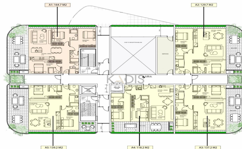
LEVEL 01 1:100
