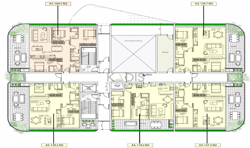
1 LEVEL 01 1:100
