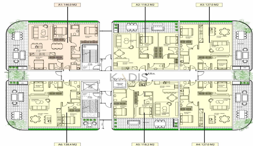
① LEVELS 02-08 1:100
