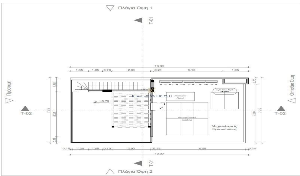
3. Κάτοψη Ταράτσας 1:100
