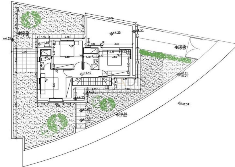
Κάτοψη ορόφου
