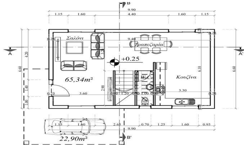
ΚΑΤΟΨΗ ΙΣΟΓΕΙΟΥ ΚΑΤΟΙΚΙΑ 1
