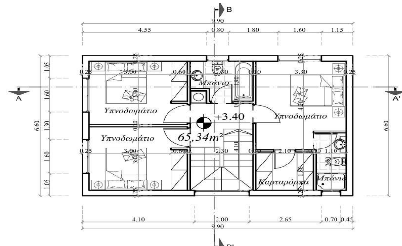
ΚΑΤΟΨΗ ΟΡΟΦΟΥ ΚΑΤΟΙΚΙΑ 1
