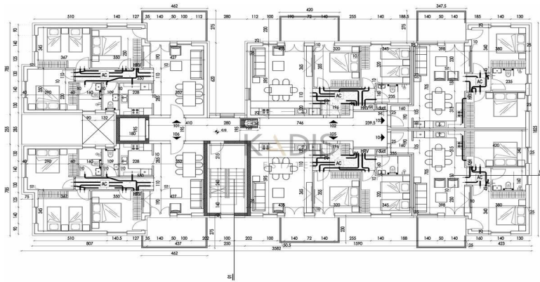
Κάτοψη ορόφου 1 1:100
