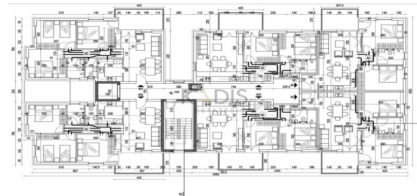
Κάτοψη ορόφου 4 1:100
