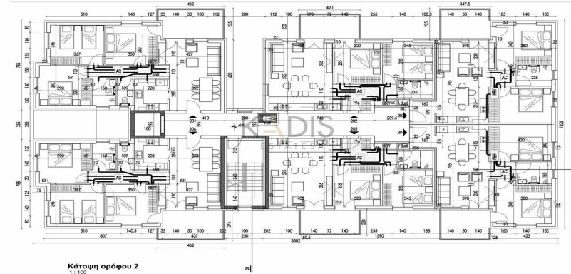
Κάτοψη ορόφου 2 1:100
