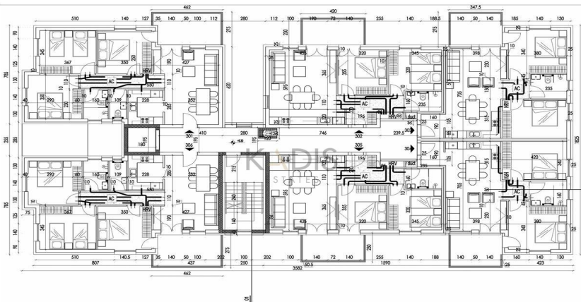
Κάτοψη ορόφου 3 1:100
