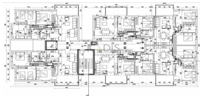
Κάτοψη ορόφου 4 1:100
