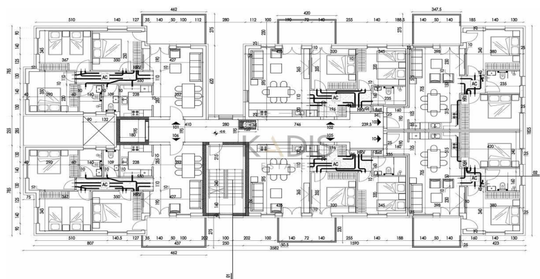
Κάτοψη ορόφου 1 1:100
