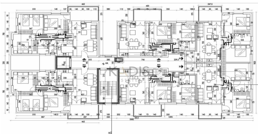
Κάτοψη ορόφου 3 1:100
