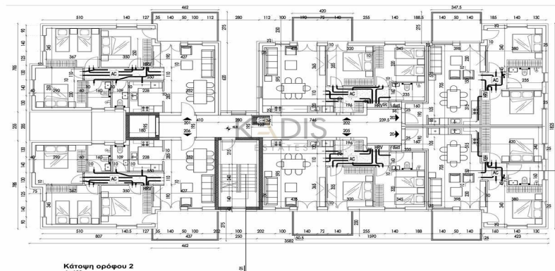
Κάτοψη ορόφου 2 1:100
