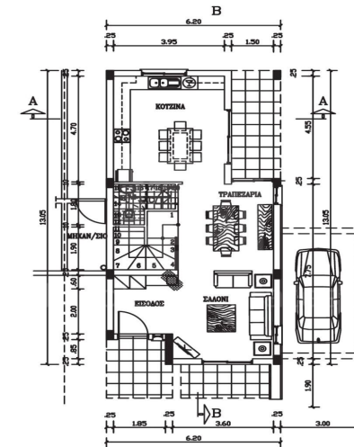
ΚΑΤΟΨΗ ΙΣΟΓΕΙΟΥ ΤΥΠΟΥ Β'
