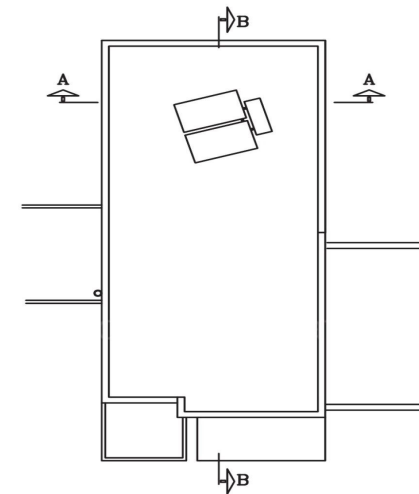
ΚΑΤΟΨΗ ΙΣΟΓΕΙΟΥ ΤΥΠΟΥ Β'
