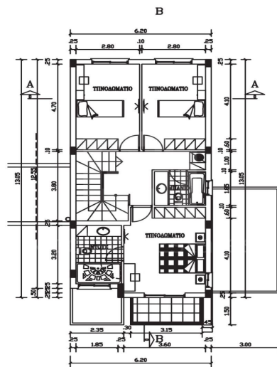
ΚΑΤΟΨΗ ΟΡΟΦΟΥ ΤΥΠΟΥ Β'
