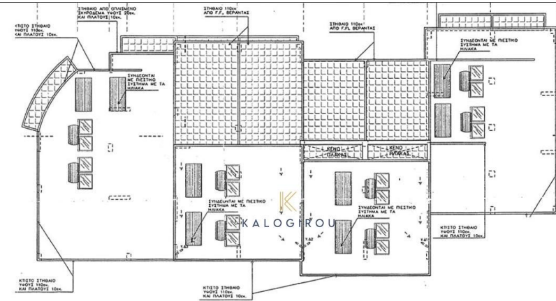
4 ΚΑΤΩΣΤΕΡΟ 4ου ΟΡΟΦΟΥ ΚΑΙΜΑΚΑ 1:100
