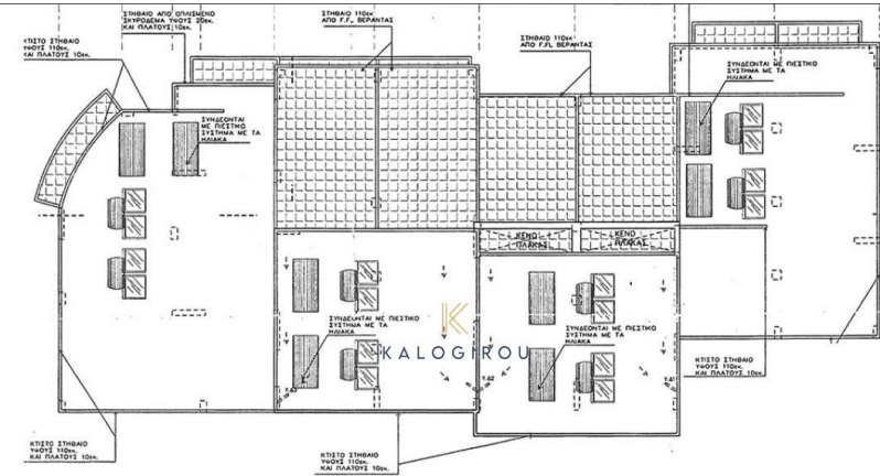
4 ΚΑΤΩΨΗΣ ΟΡΟΦΗΣ ΚΑΙΜΑΚΑ 1:100
