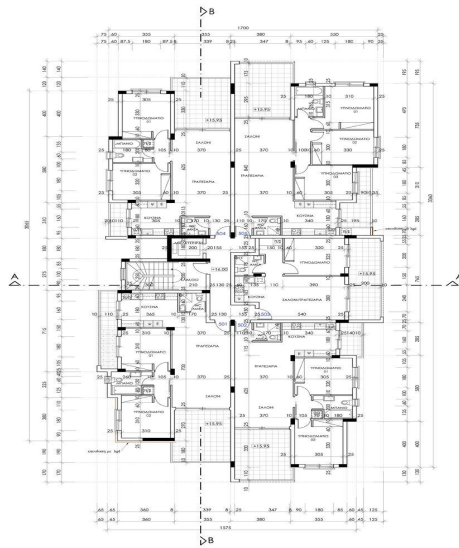
ΚΑΤΩΦΙ ΓΕΜΠΛΟΥ ΟΡΟΦΟΥ ΠΟΛΥΚΑΤΟΙΚΙΑ BLOCK A
