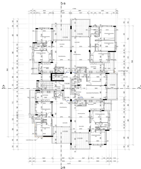
ΚΑΤΩΦΗ ΓΕΜΠΛΟΥ ΟΡΟΦΟΥ ΠΟΛΥΚΑΤΟΙΚΙΑ BLOCK A
