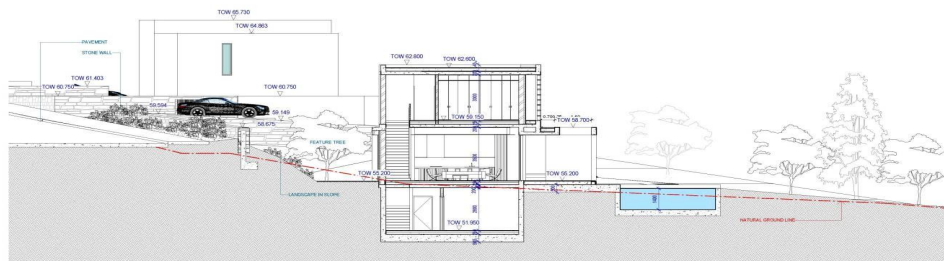
1 PLOT 02_Section 01 SCALE: 1 : 100
