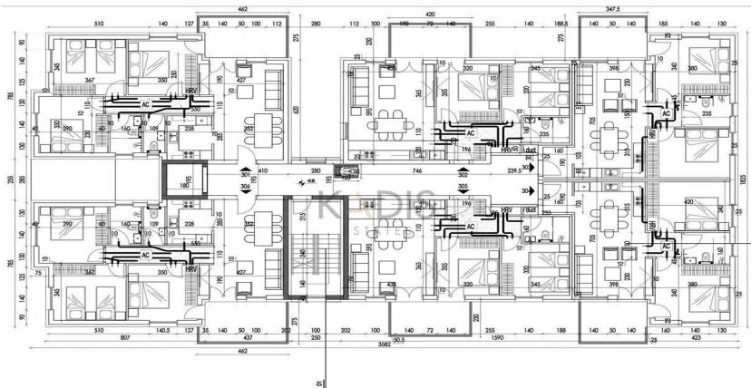
Κάτοψη ορόφου 3 1 : 100
