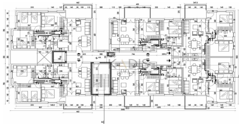
Κάτοψη ορόφου 1 1 : 100
