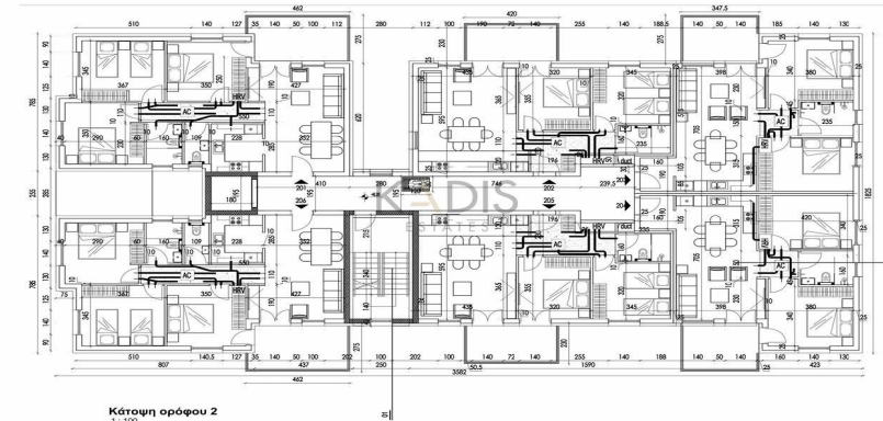
Κάτοψη ορόφου 2 1 : 100
