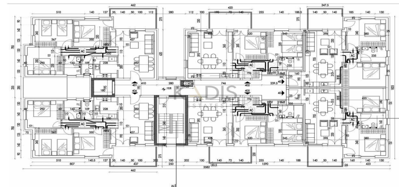
Κάτοψη ορόφου 4 1 : 100
