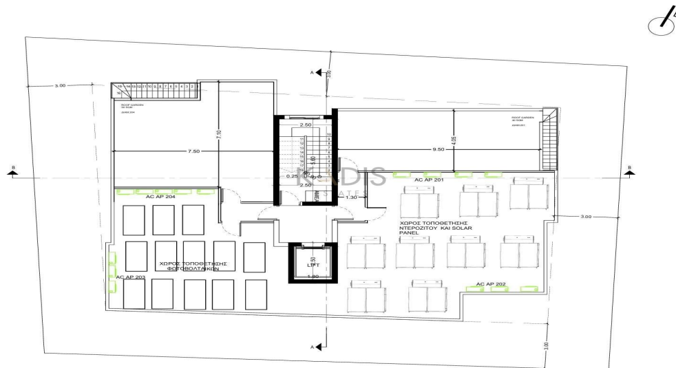
ΚΑΤΟΨΗ ΟΡΟΦΗΣ
