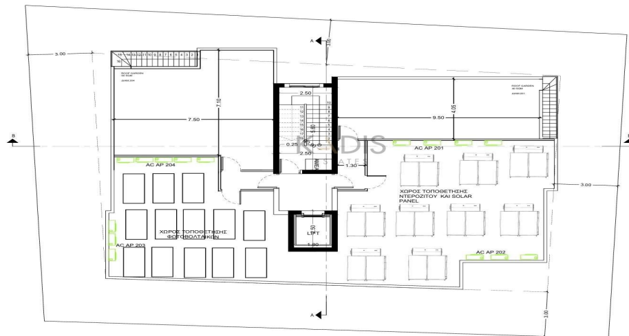
ΚΑΤΟΨΗ ΟΡΟΦΗΣ
