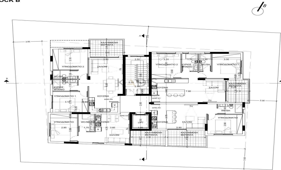
ΚΑΤΟΨΗ 1ΟΥ ΟΡΟΦΟΥ
