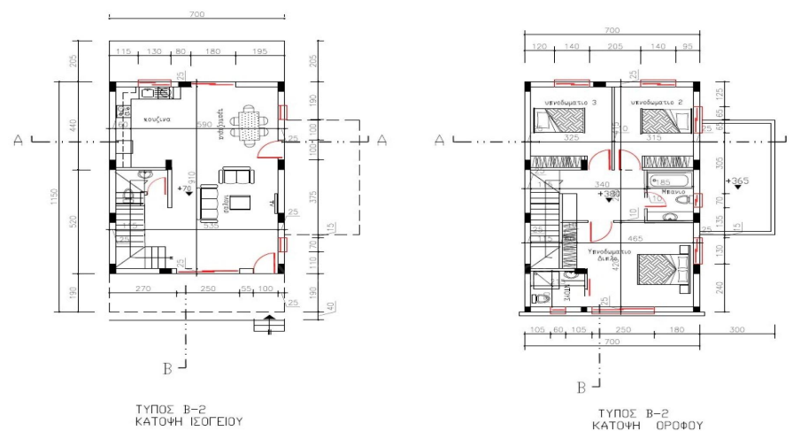
ΤΥΠΟΣ Β-2 - ΟΙΚΙΑ 5
