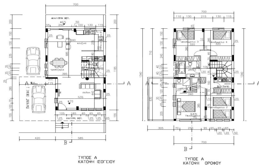
ΤΥΠΟΣ Α - ΟΙΚΙΕΣ 1, 4
