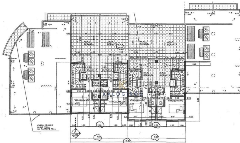
3) ΚΑΤΩΦΗΣ 2ου ΟΡΟΦΟΥ ΚΑΙΜΑΚΑ 1:100
