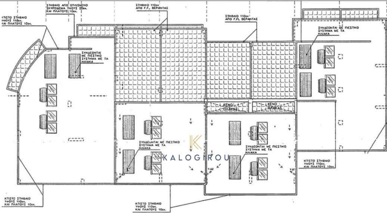
4) ΚΑΤΩΨΗΣ 4ου ΟΡΟΦΟΥ ΚΑΙΜΑΚΑ 1:100
