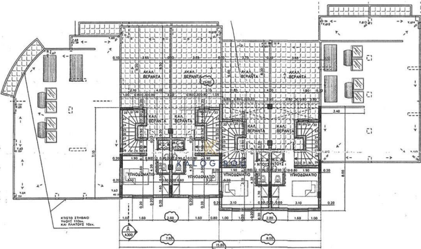
3) ΚΑΤΩΨΗΣ 2ου ΟΡΟΦΟΥ ΚΑΙΜΑΚΑ 1:100
