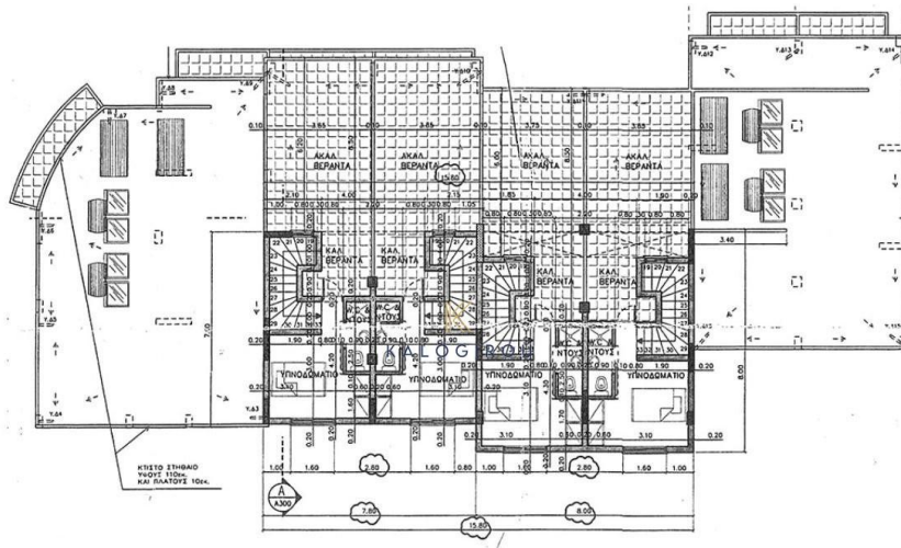
3) ΚΑΤΩΦΗΣ 3ου ΟΡΟΦΟΥ ΚΑΙΜΑΚΑ 1:100
