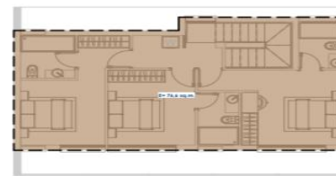
④ AREA PLAN F.F. 1 : 100
