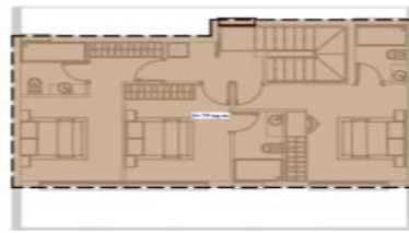
④ AREA PLAN F.F. 1 : 100
