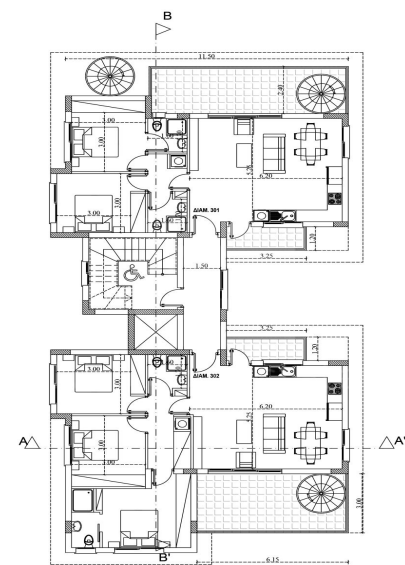
ΚΑΤΟΨΗ 3ου ΟΡΟΦΟΥ
