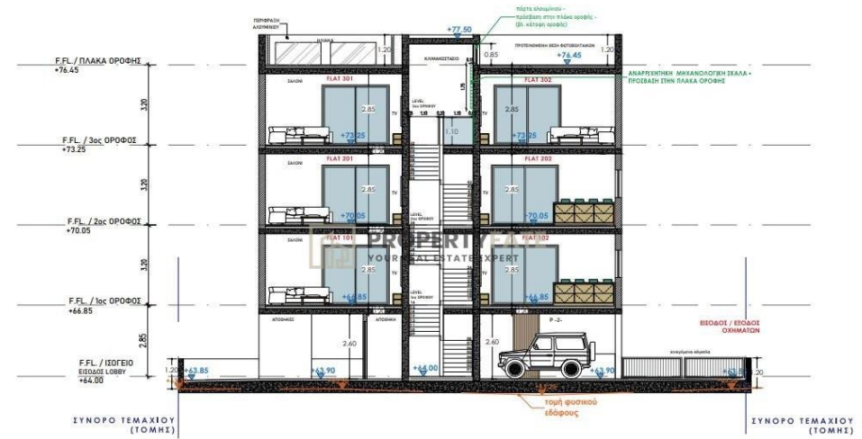
ΤΟΜΗ BB
