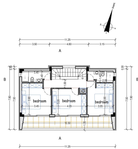
κατοψη οροφου
