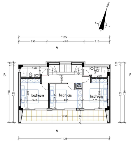
κατοψη οροφου
