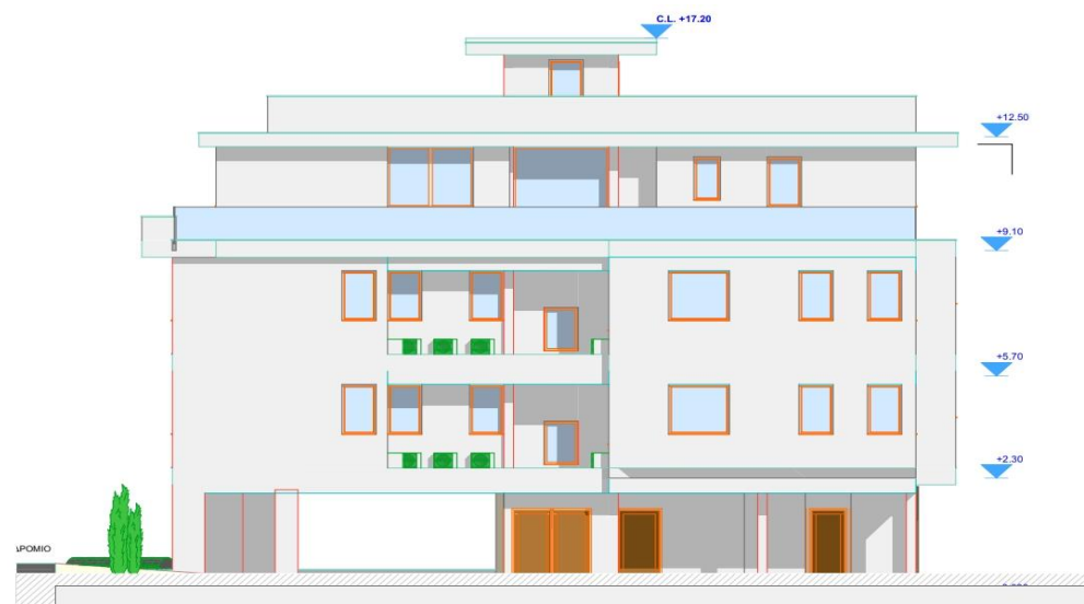
ΑΝΑΤΟΛΙΚΗ ΟΨΗ 1:100
