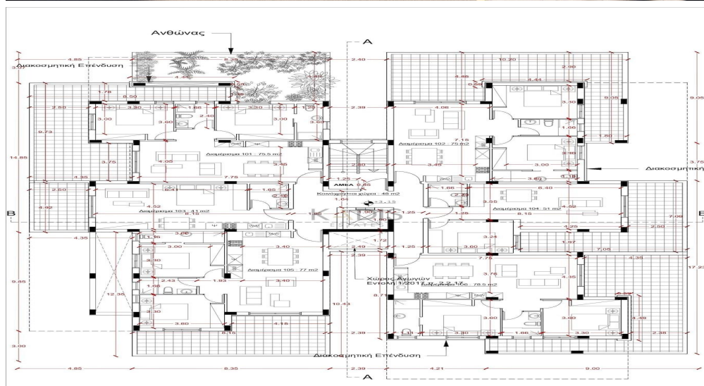
Κάτοψη 1ου Ορόφου
