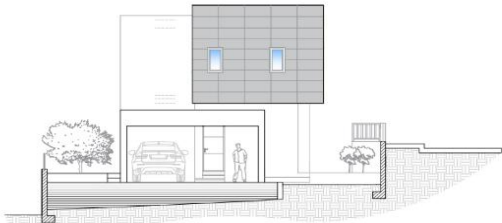
ΠΛΑΓΙΑ ΟΨΗ ΚΑΤΟΙΚΙΑ "A"
