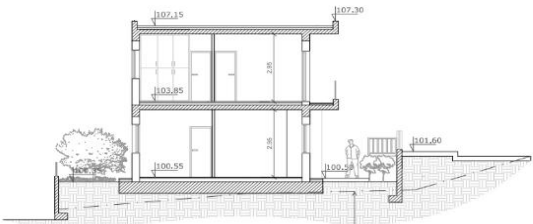
ΤΟΜΗ Β - Β
