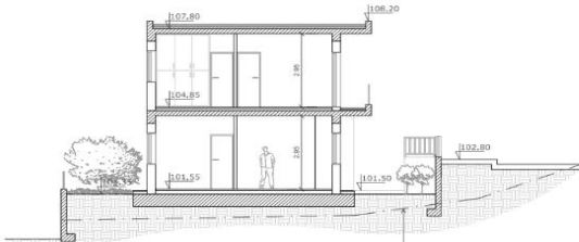
ΤΟΜΗ Γ - Γ
