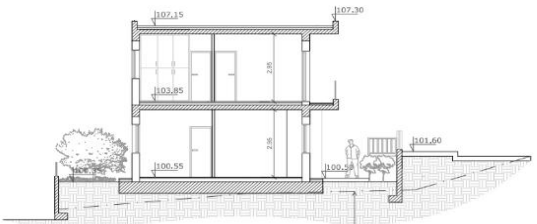
ΤΟΜΗ Β - Β
