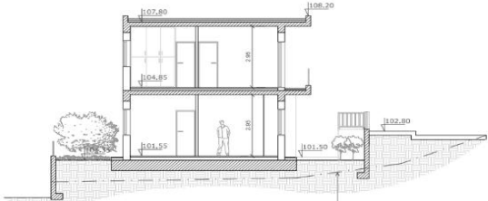
ΤΟΜΗ Γ - Γ
