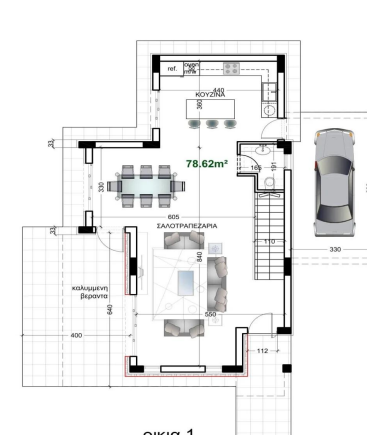
οικία 1 κατοψη ισογειου κλίμακα 1 : 100
