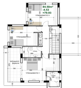
οικια 1 κατοψη 1ου οροφου κλίμακα 1 : 100
