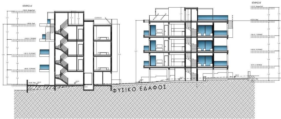
ΤΟΜΗ Α - Α ΚΛΙΜΑΚΑ 1/200
