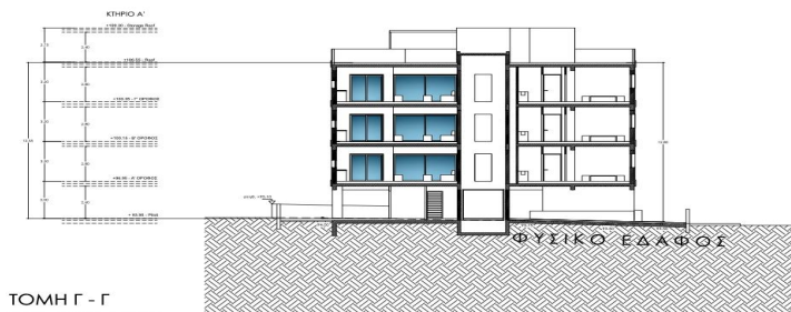
ΤΟΜΗ Γ - Γ ΚΛΙΜΑΚΑ 1/200
