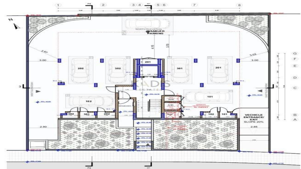
ΧΩΡΟΤΑΞΙΚΟ - ΙΣΟΓΕΙΟ ΚΑΙΜΑΚΑ 1:200
