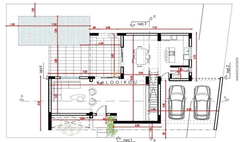
τεμάχιο 14 / κάτοψη ισογείου
