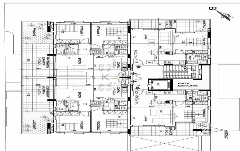
1ος ΟΡΟΦΟΣ
