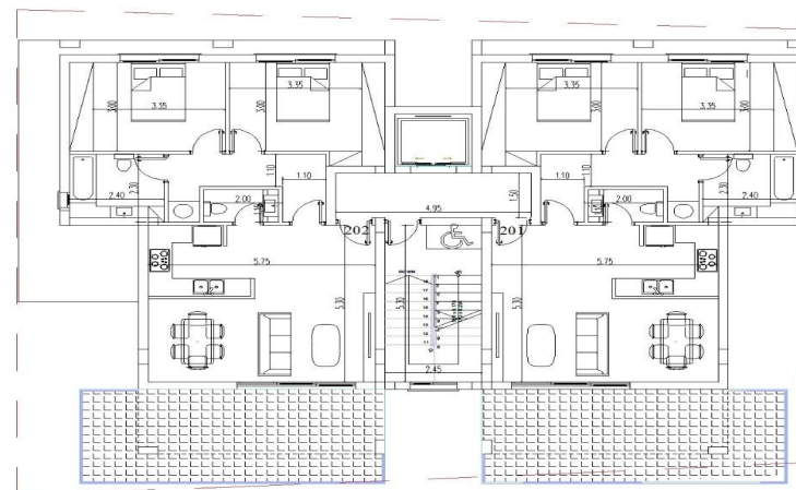
ΚΑΤΟΨΗ 2ου ΟΡΟΦΟΥ
