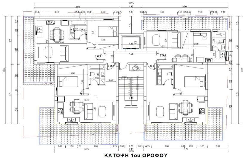
ΚΑΤΟΨΗ 1ου ΟΡΟΦΟΥ
