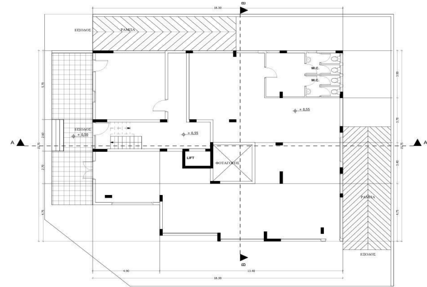
ΚΑΤΟΨΙΣ ΚΑΤΑΣΤΗΜΑΤΩΝ
