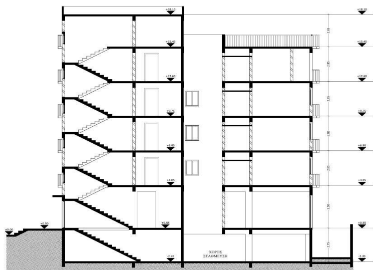
ΤΟΜΗ Α-Α
