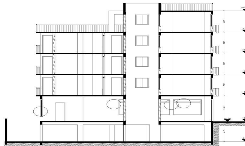
ΤΟΜΗ Β-Β
