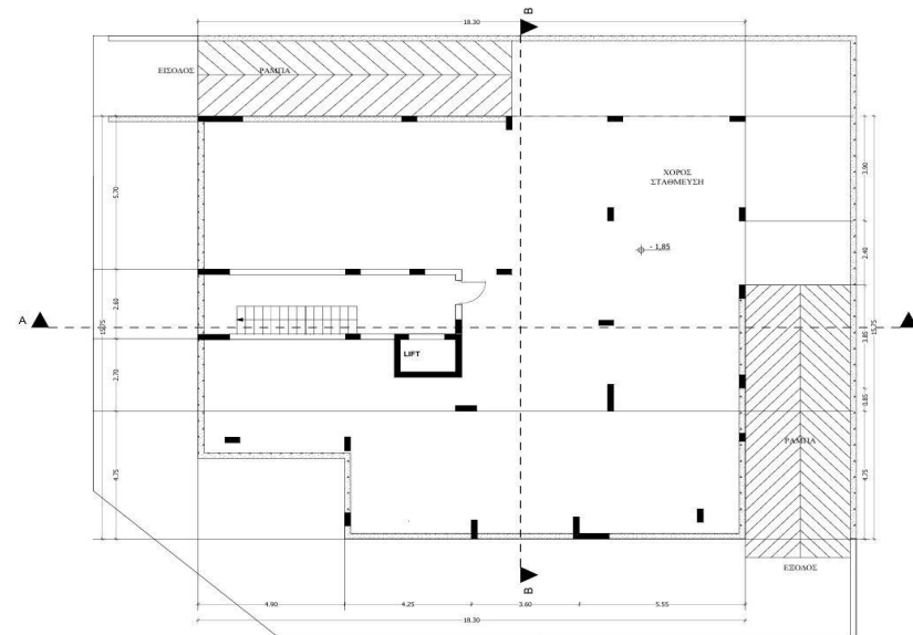
ΚΑΤΟΨΙΣ ΥΠΟΣΤΕΓΟΥ
