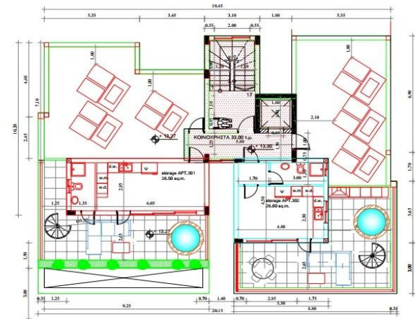
ΚΑΤΟΨΗ ROOF GARDEN
