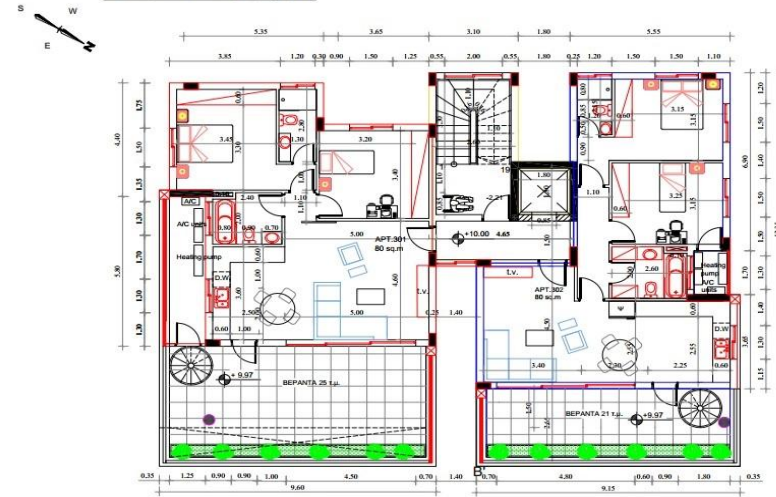
ΚΑΤΟΨΗ Γ' ΟΡΟΦΟΥ
