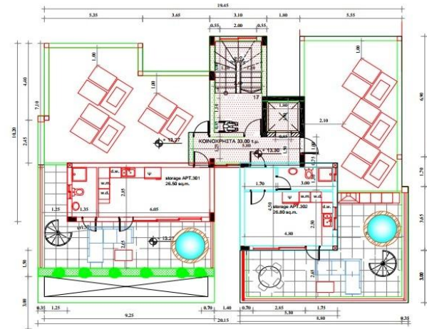
ΚΑΤΟΨΗ ROOF GARDEN
