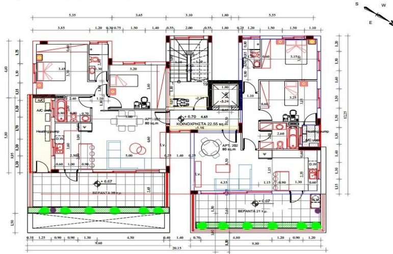
ΚΑΤΟΨΗ Β' ΟΡΟΦΟΥ
