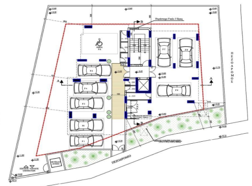
ΚΑΤΟΠΗ ΙΣΟΓΕΙΟΥ (ΧΩΡΟΤΑΞΙΚΟ)
