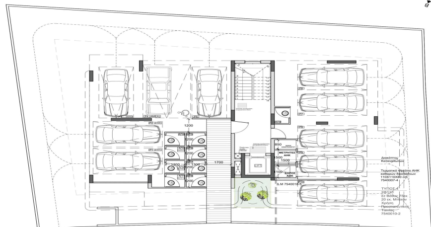
ΚΑΤΟΨΗ ΙΣΟΓΕΙΟΥ
