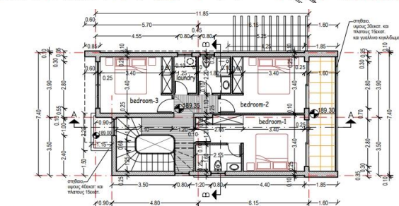
κατομή ορόφου επώλη 19 Εμβανα = 84,541 μ. - 12,291 μ. = 72,250 μ. Εκλ.δω.ορ. = 11,041 μ.
