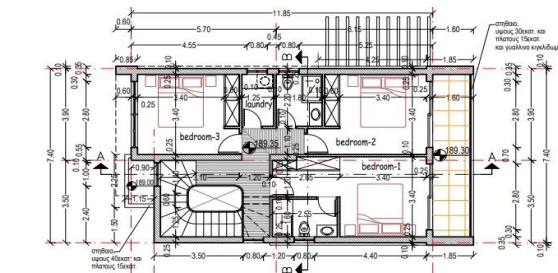
κατοψη οροφου επταλη 19
