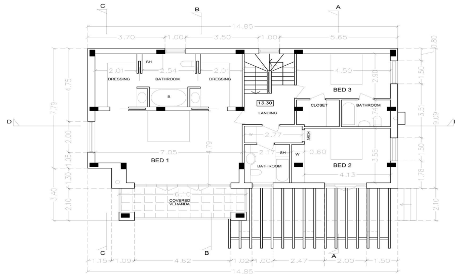
ΤΕΛΙΚΗ ΚΑΤΟΨΗ ΟΡΟΦΟΥ
