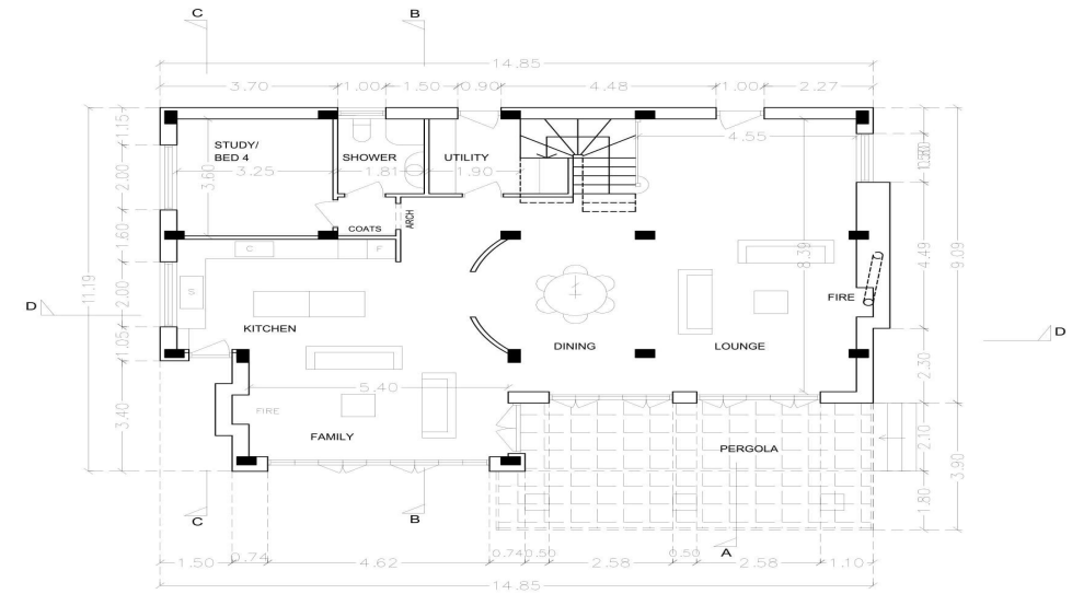
ΤΕΛΙΚΗ ΚΑΤΟΨΗ ΙΣΟΓΕΙΟΥ
