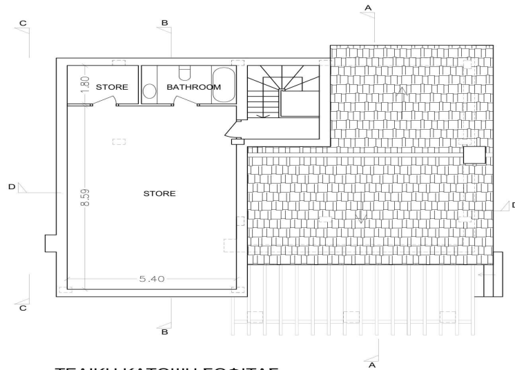
ΤΕΛΙΚΗ ΚΑΤΟΨΗ ΣΟΦΙΤΑΣ
