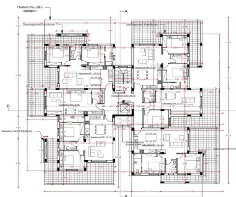
Κάτοψη 3ου Ορόφου
