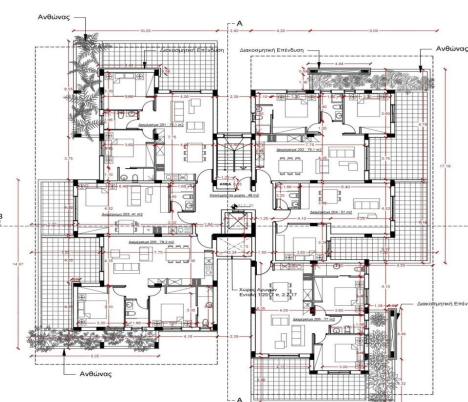
Κάτοψη 4ου Ορόφου
