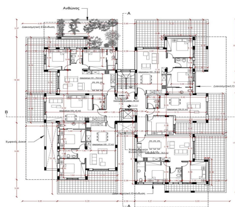
Κάτοψη 1ου Ορόφου
