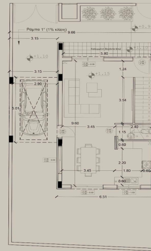
ΚΑΤΟΨΗ ΙΣΟΓΕΙΟΥ
