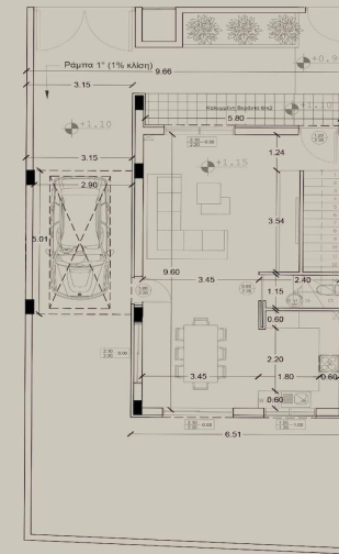
ΚΑΤΟΨΗ ΙΣΟΓΕΙΟΥ
