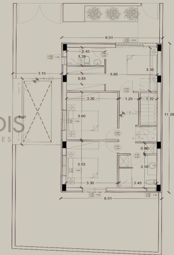
ΚΑΤΟΨΗ ΟΡΟΦΟΥ
