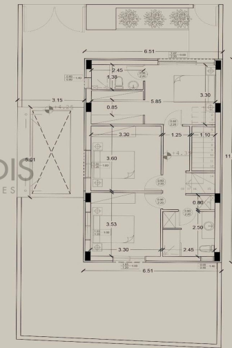
ΚΑΤΟΨΗ ΟΡΟΦΟΥ
