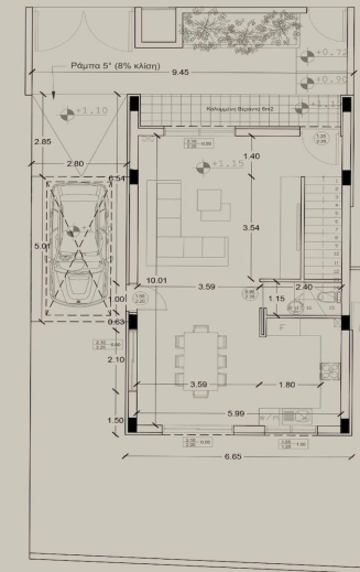
ΚΑΤΟΨΗ ΙΣΟΓΕΙΟΥ
