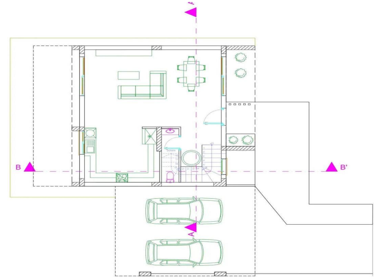
ΚΑΤΩΦΗ ΙΣΟΓΕΙΟΥ
