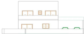
ΔΥΤΙΚΗ ΟΨΗ
