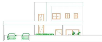
ΑΝΑΤΟΛΙΚΗ ΟΨΗ
